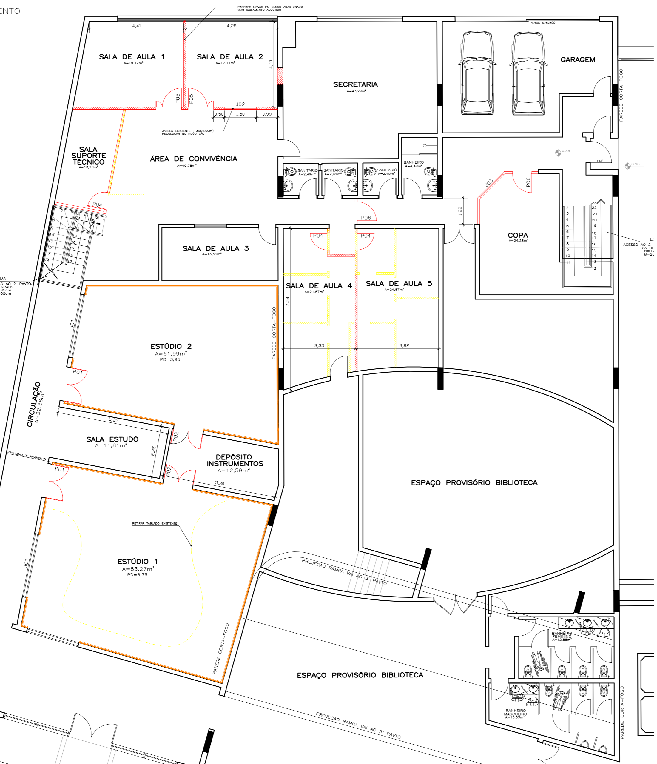
PLANTA BAIXA - TÉRREO ESC.:1/100
