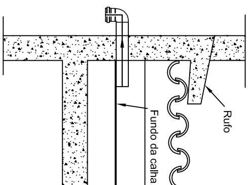
Detalhe 09 - Extravassor da Calha Escala 1:20
